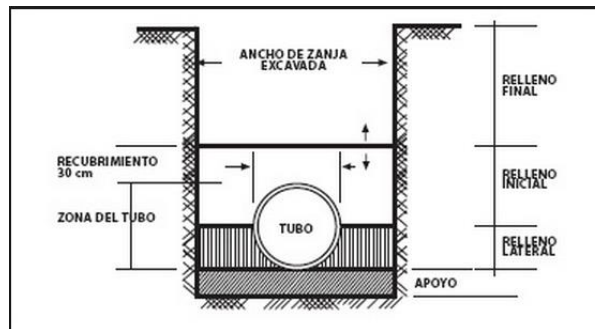
Figura. Dimensiones de excavación
