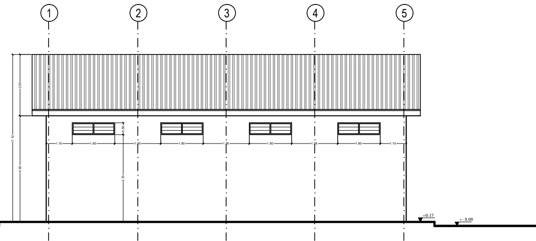
ELEVACIÓN LATERAL ESC. 1:150
