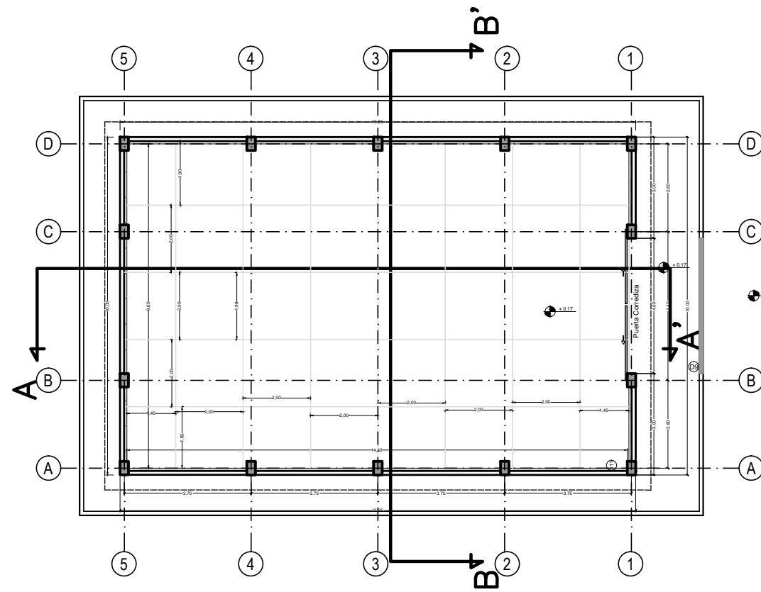
PLANTA GALPÓN ESC. 1:150
