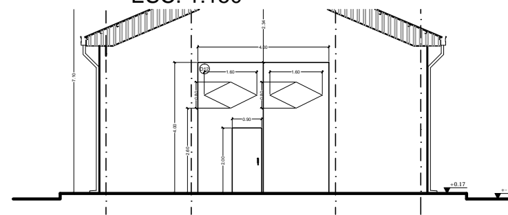
ELEVACIÓN POSTERIOR ESC. 1:150
