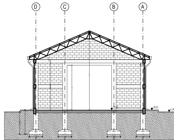
CORTE B-B' ESC. 1:150
