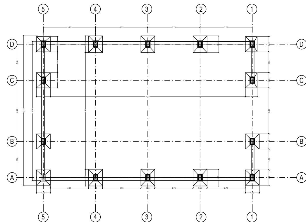
PLANO DE CIMIENTOS ESC. 1:150
