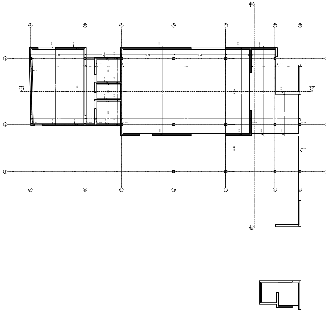
PLANO DE CIMIENTOS ESC. 1: 75
