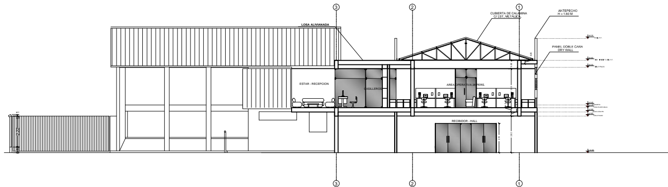
CORTE B - B ESC. 1: 75
