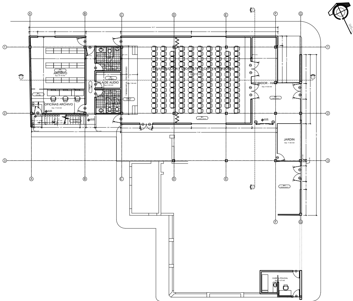
PLANTA BAJA ESC. 1: 75
