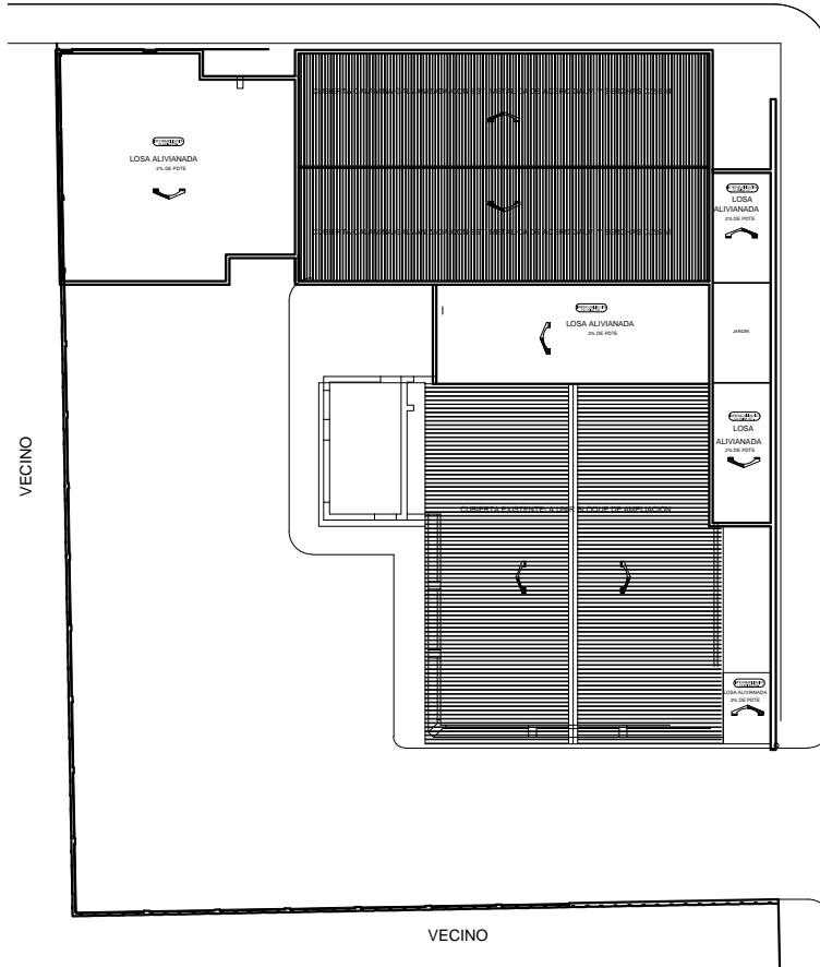
PLANO DE SITIO Y TECHOS ESC. 1:75
