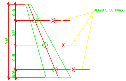
DETALLE 7 ESC. 1:5
