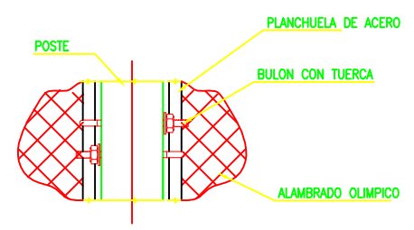
DETALLE 9 ESC. 1:5
