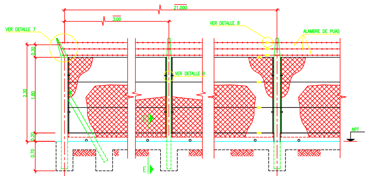
ELEVACION TIPICA DE CERCA ESCALA 1:25
