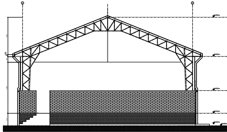
ELEVACION LATERAL IZQUIERDA ESC.: 1 : 50
