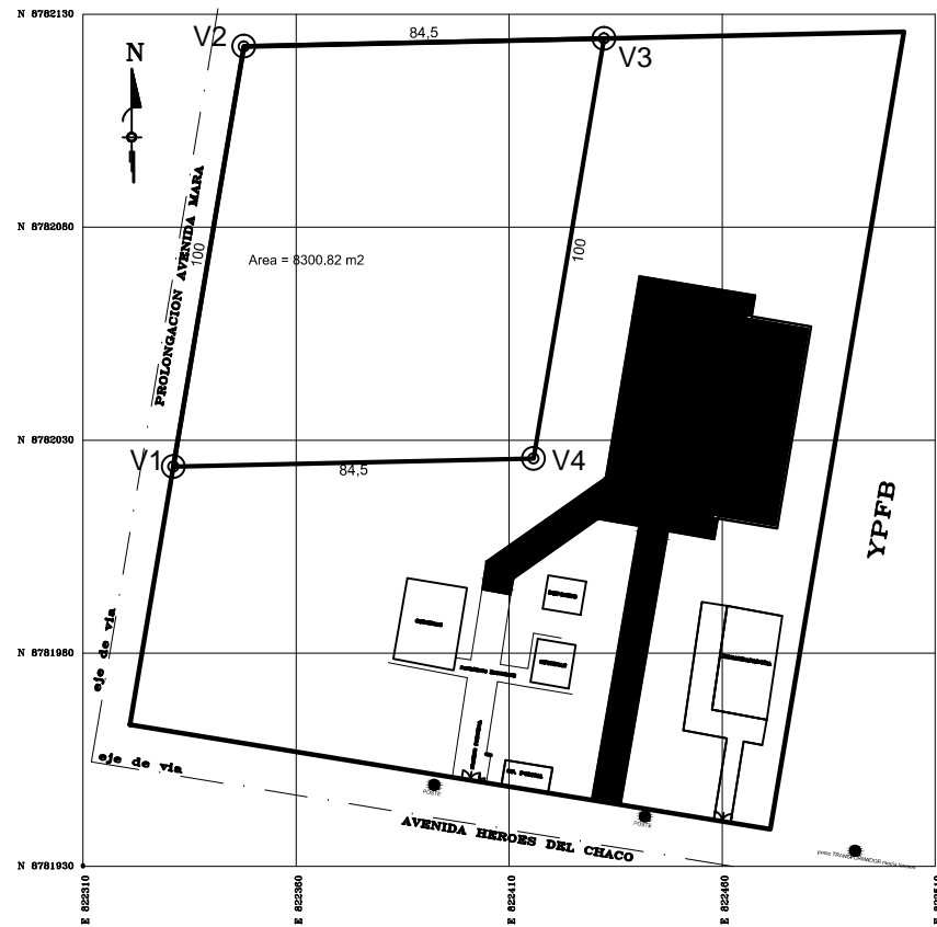
UBICACION EN SITIO ESC.: 1 : 500
