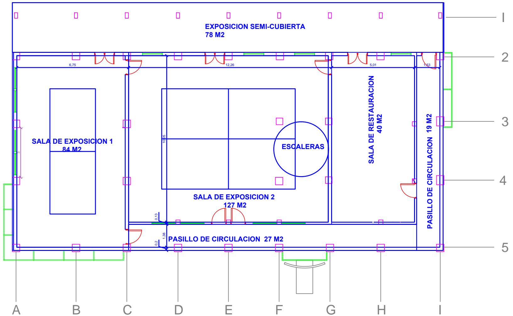
PLANTA ALTA
