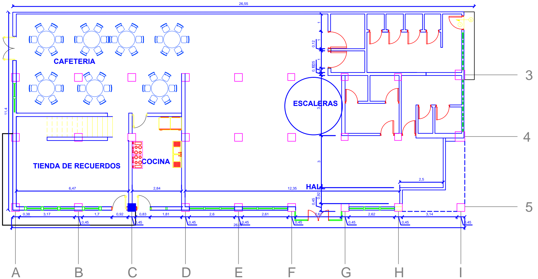
PLANTA BAJA
