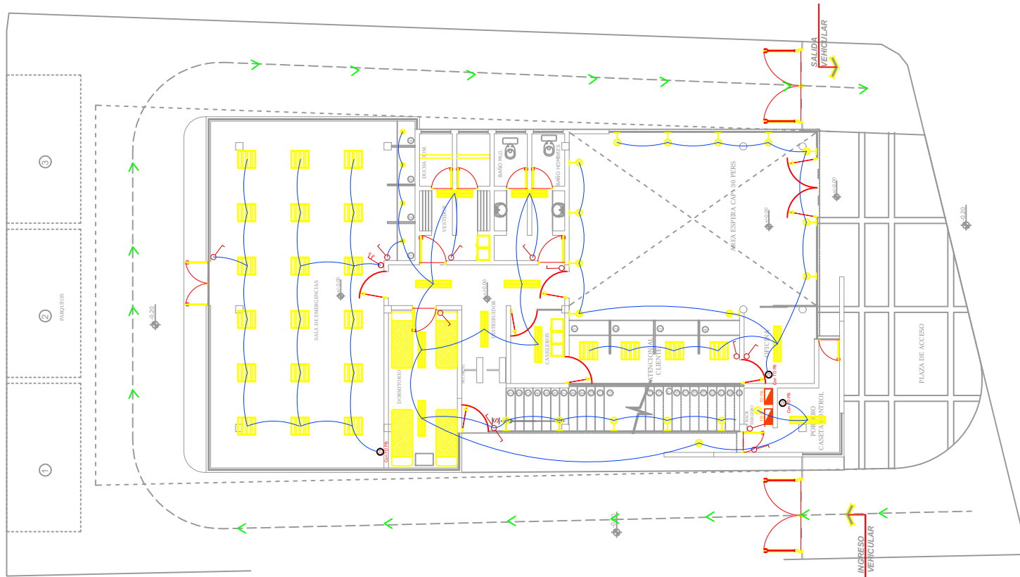
PLANO PLANTA BAJA ESC. : 1 : 50
