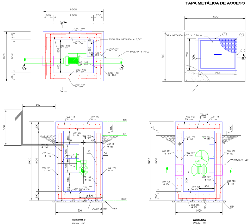
ELEVACION B (ESCALA 1:25)
