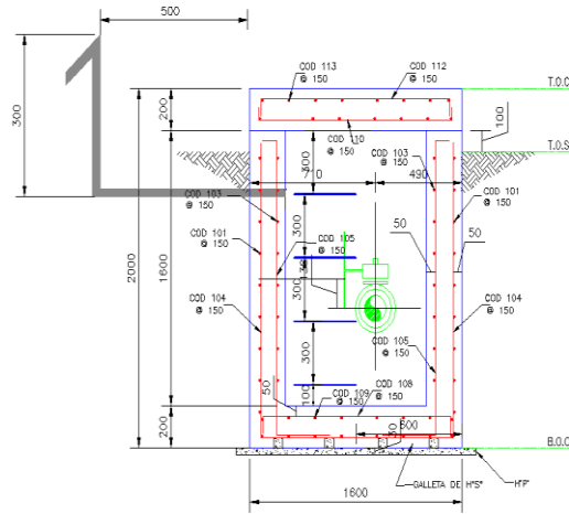
ELEVACION A (ESCALA 1:25)
