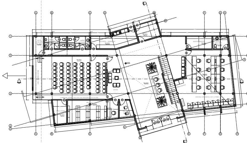
PLANTA BAJA ESL: 1:100 OFICINAS DISTRITO COMERCIAL AMAZONICO - RIBERALTA
