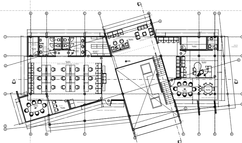
PLANTA ALTA ESL: 1:100 OFICINAS DISTRITO COMERCIAL AMAZONICO - RIBERALTA
