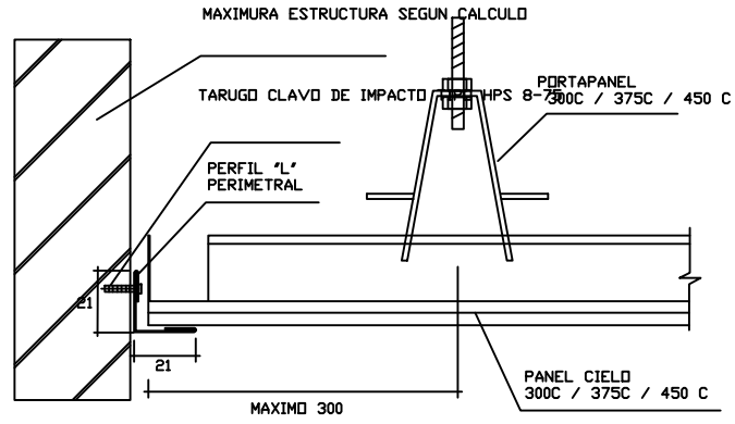
REMATE PERFIL "L"
