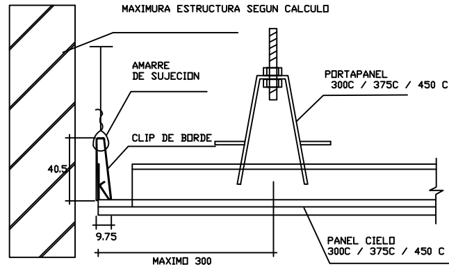
REMATE PERFIL DE BORDE
