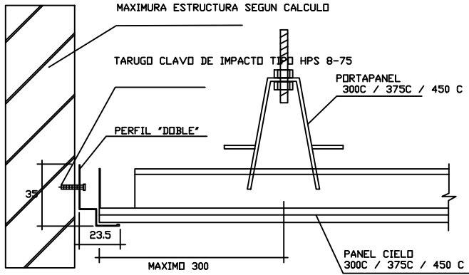
REMATE PERFIL DOBLE "L"
