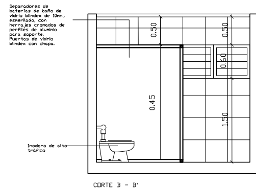
PLANO DE CORTES Y ELEVACIONES
