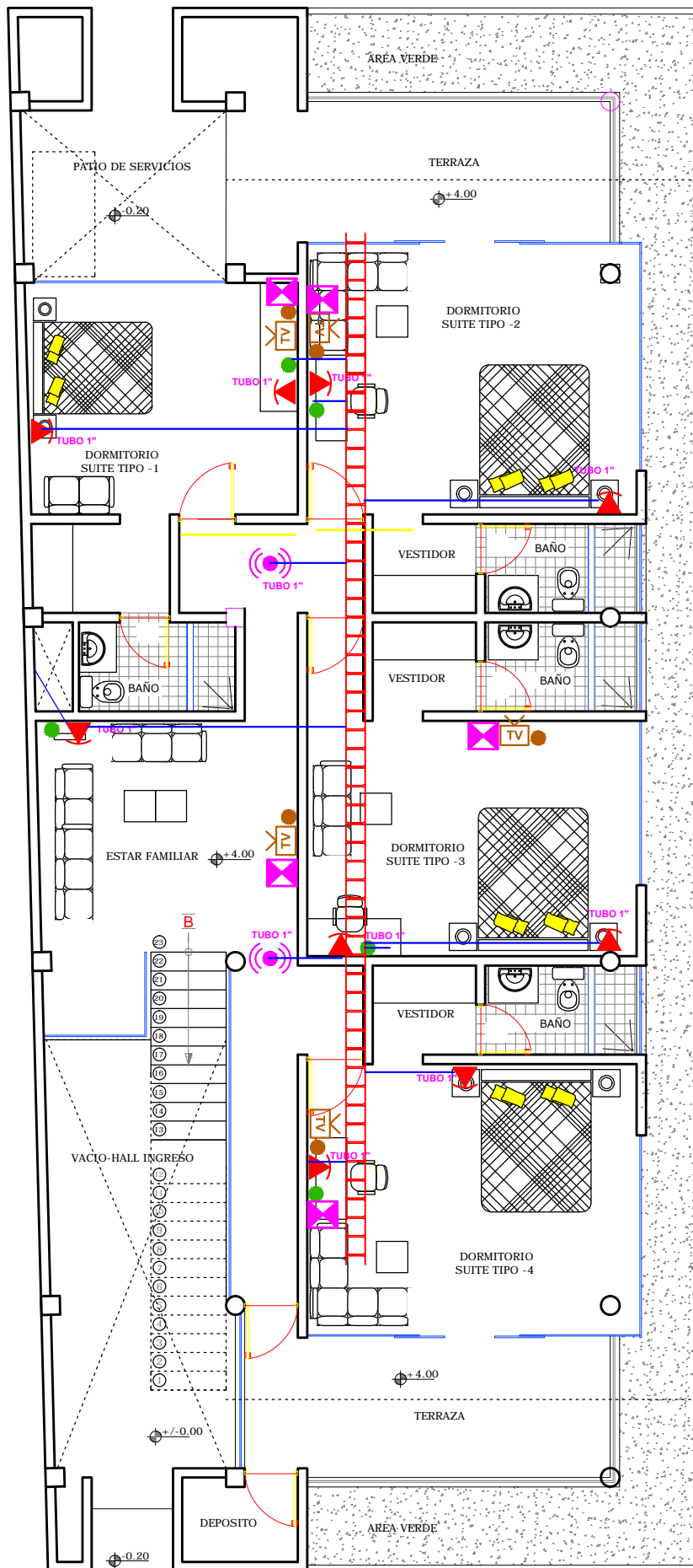
PLANO PLANTA ALTA
