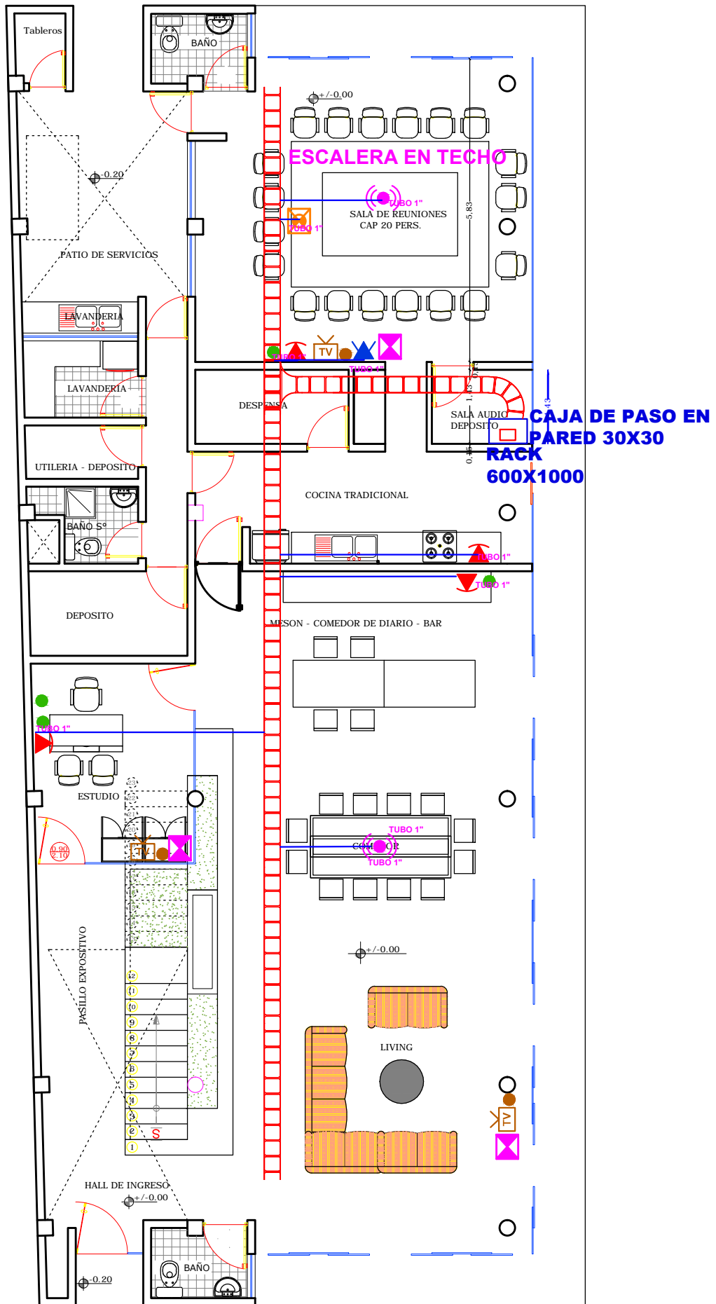
PLANO PLANTA BAJA
