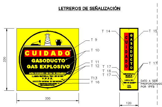
PLANILLA 1 TAMAÑOS DE LETRAS LETREROS DE SEÑALIZACIÓN
