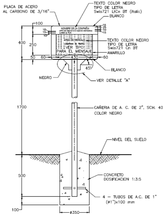
ELEVACION
