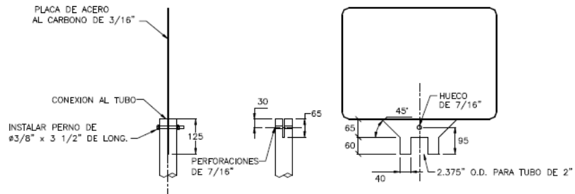
DETALLE "A"
