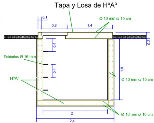
ELEVACIÓN
