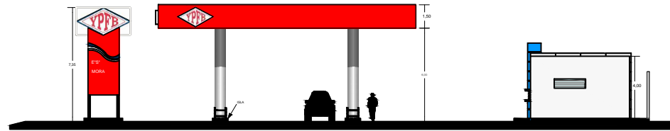
ELEVACION LATERAL DERECHO EN CONJUNTO
