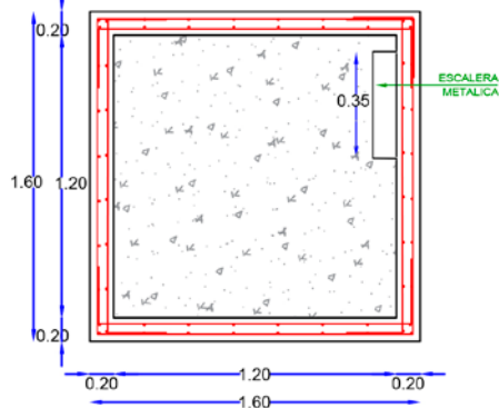
CÁMARA DE HºAº VISTA EN PLANTA
