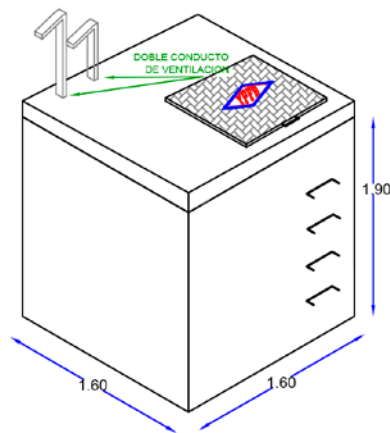
VISTA EN ELEVACION ISOMETRICA
