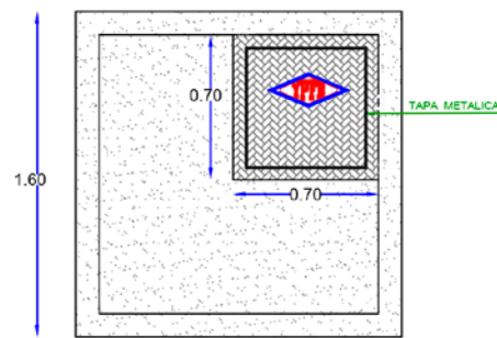
TAPA METALICA DE ACCESO VISTA EN PLANTA
