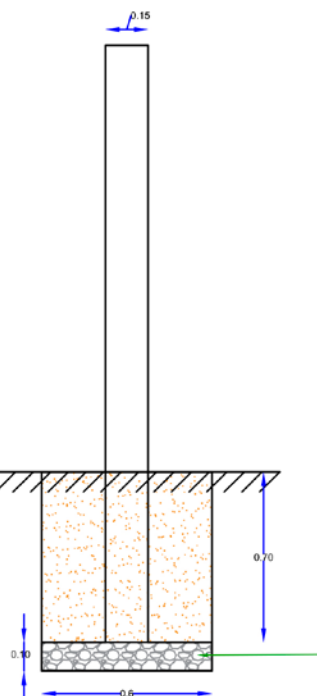
DETALLE DE VACIADO DE H o C o PARA EL PLANTADO DE LOS POSTES
