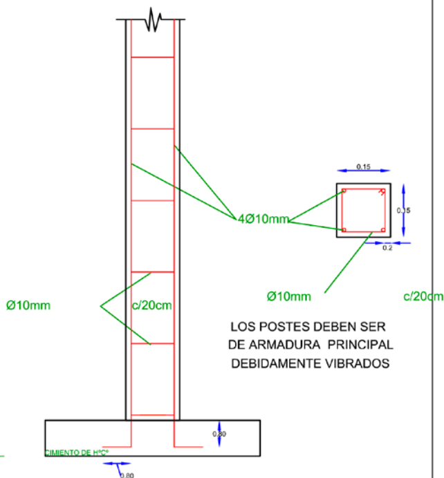
POSTE DE HORMIGÓN ARMADO (HºAº)
