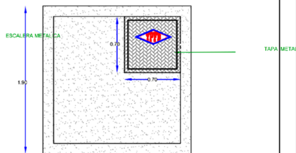
TAPA METALICA DE ACCESO VISTA EN PLANTA
