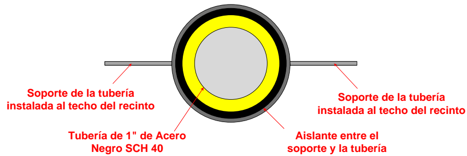
VISTA DE PLANTA
