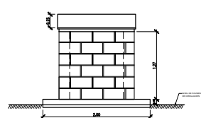
ELEVACIÓN SISTEMA DE BOMBEO ESC 1:50
