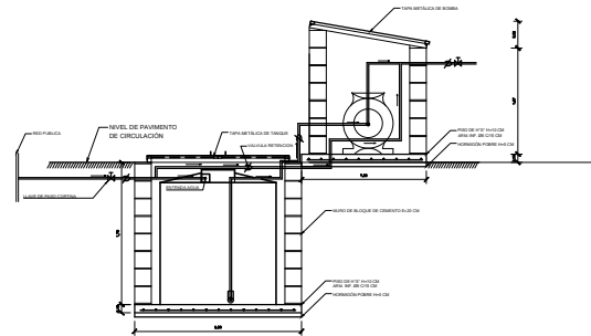
SECCION A-A' ESC 1:50
