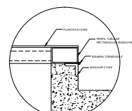
DETALLE ASENTAMIENTO Y BISAGRA DE TAPA MET. ESC 1:5
