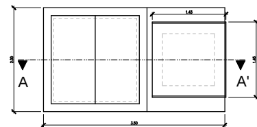
PLANTA SISTEMA DE BOMBEO ESC 1:50
