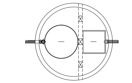
POZO SÉPTICO ABSORBENTE D=1,5 M ESC 1:25
