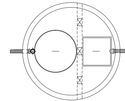
POZO SÉPTICO ABSORBENTE D=2,0 M ESC 1:25
