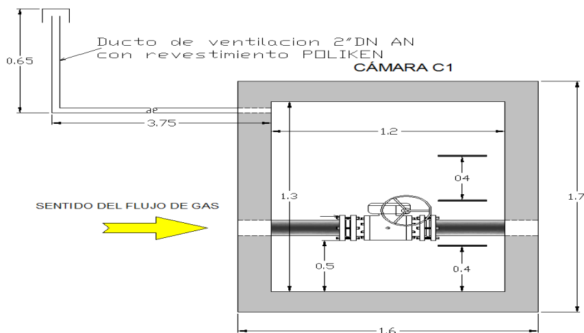
Figura 2 (vista de perfil) Interior de cámara. Estribos y ducto de ventilación.
