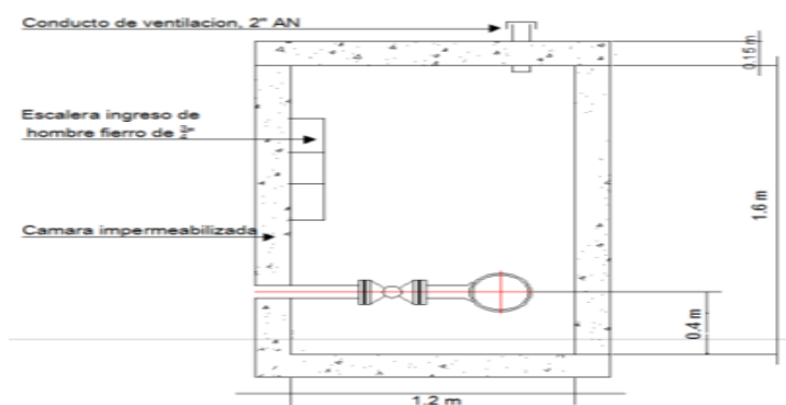
Figura 2 (vista de perfil) Interior de cámara. Estribos y ducto de ventilación.
