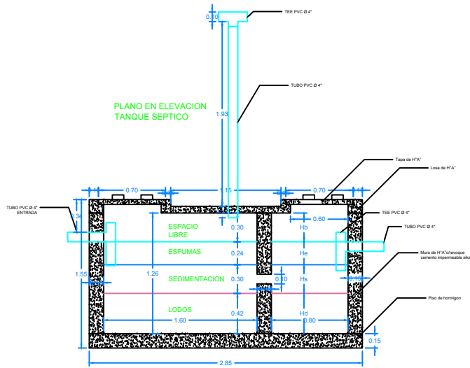
ESC. 1:50
