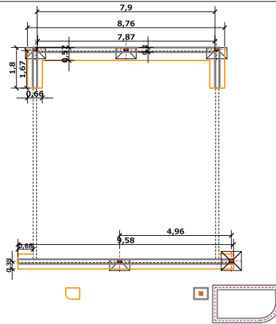
PLANO DE FUNDACIONES
