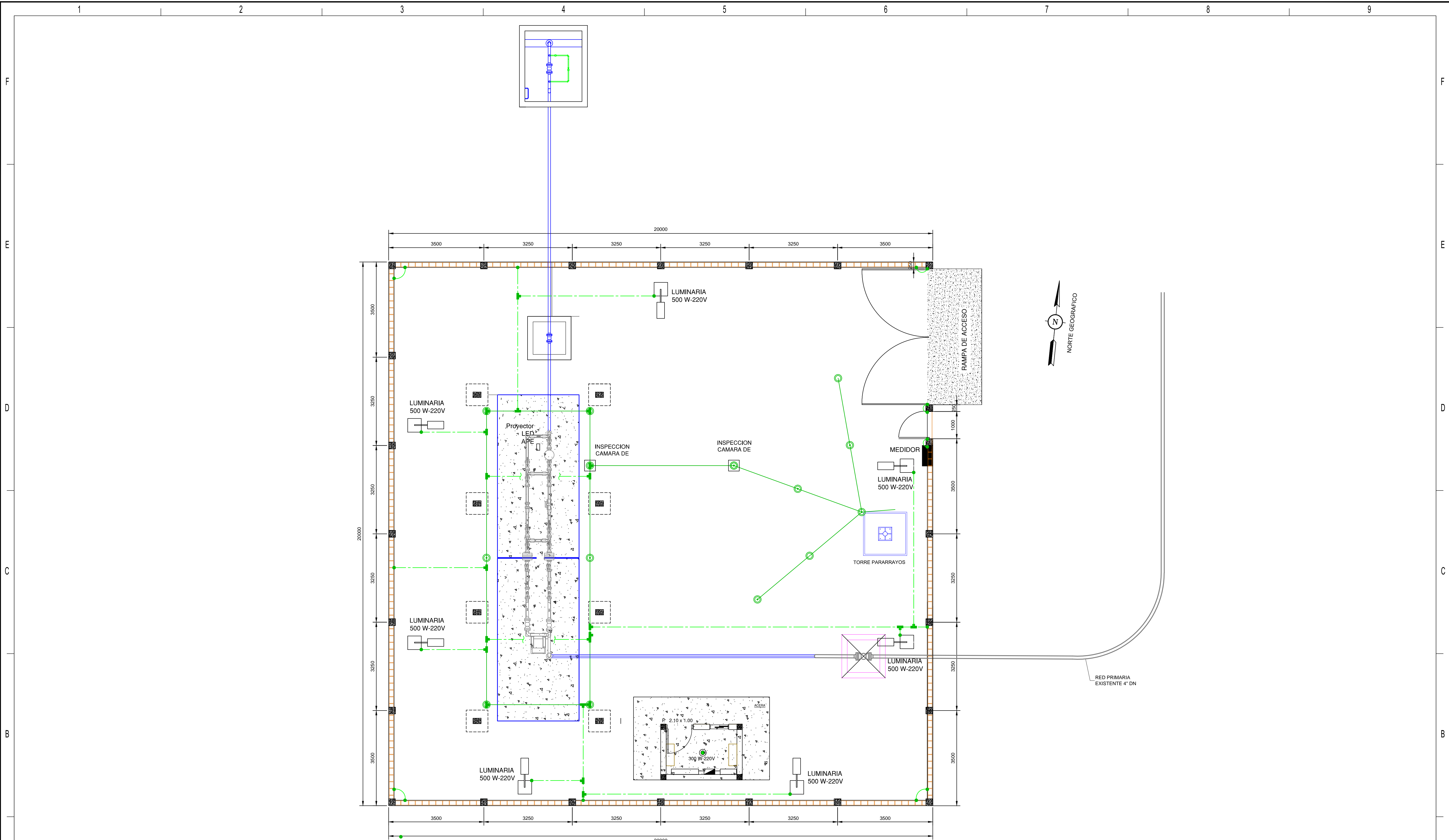
PLANO VISTA EN PLANTA CITY GATE PULQUINA BAJO
