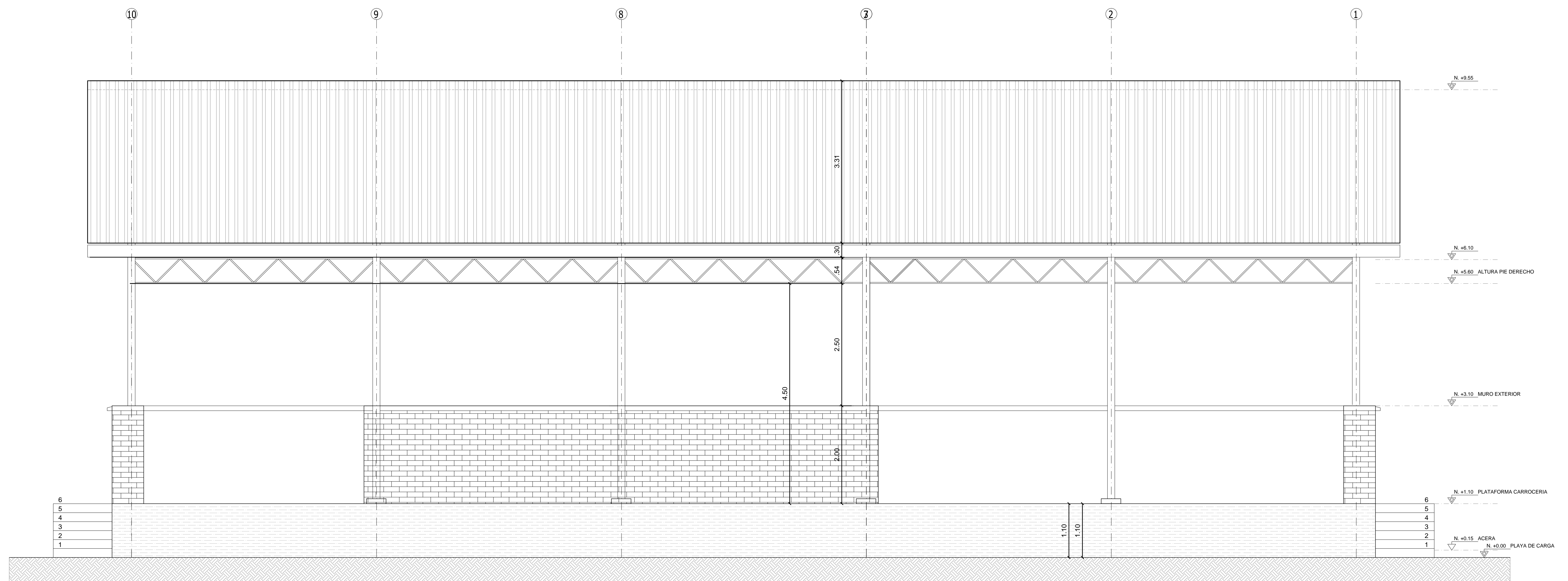
ELEVACION FRONTAL ESC. : 1 : 100
