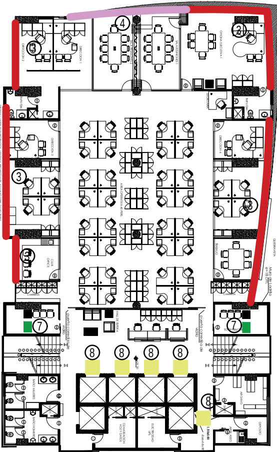
NIVEL 6-15 - OFICINAS TIPO
