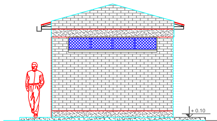
ELEV. LATERAL Escala: 1=50
