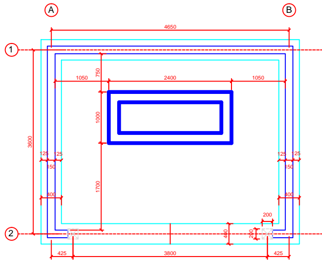
CIMENTOS Escala: 1=30
