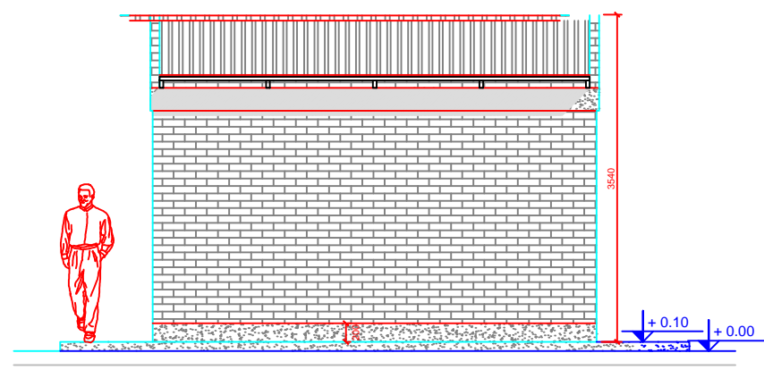
ELEV. POSTERIOR
