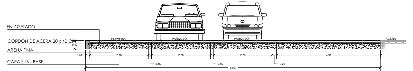
SECCIÓN A-A' ESC. 1:50
