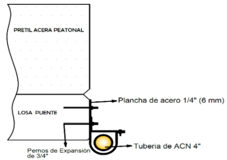
VISTA LATERAL
