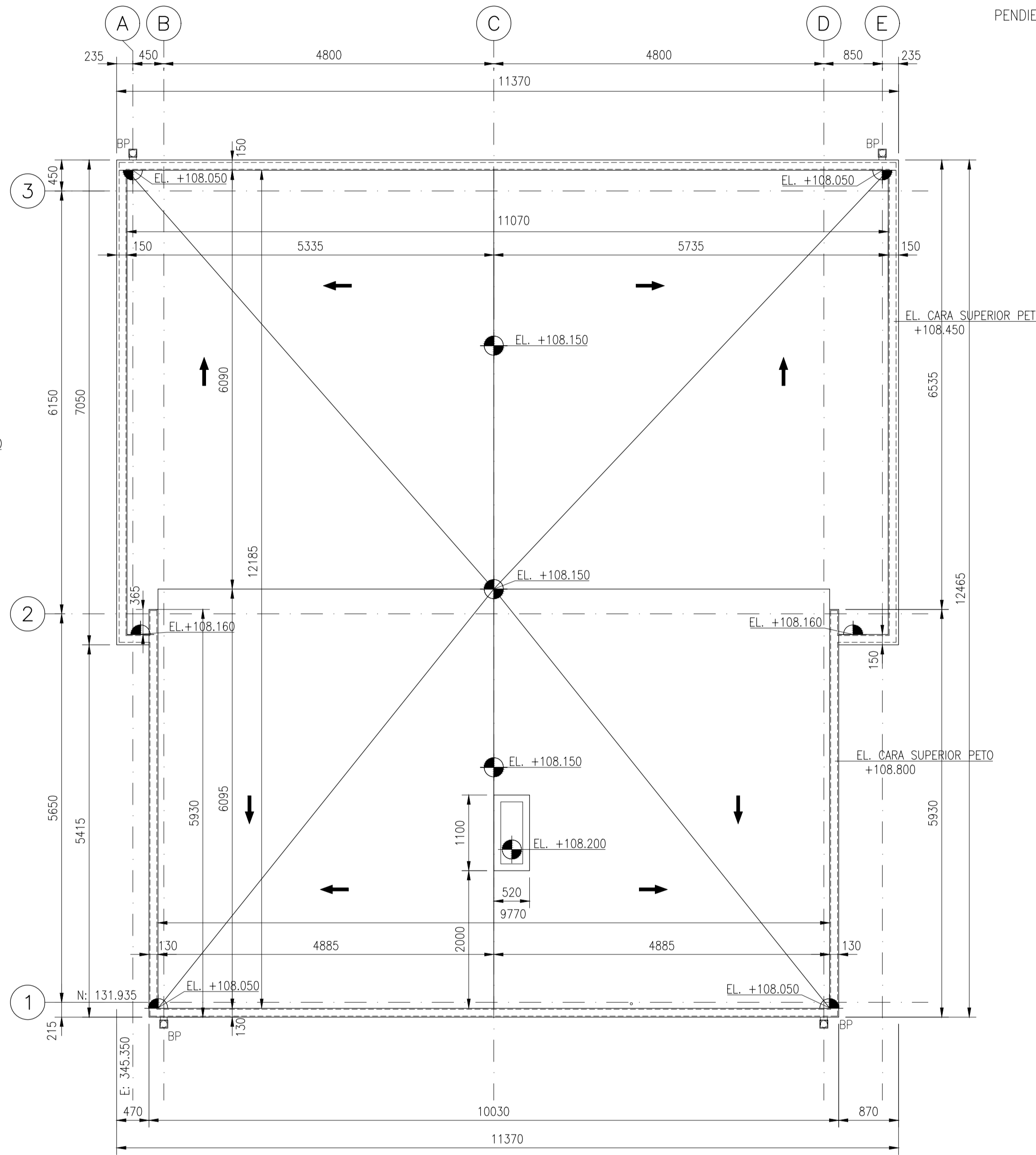
PLANTA CUBIERTA ELEVACIÓN+108.000 N.S.LOSA ESCALA 1:50
