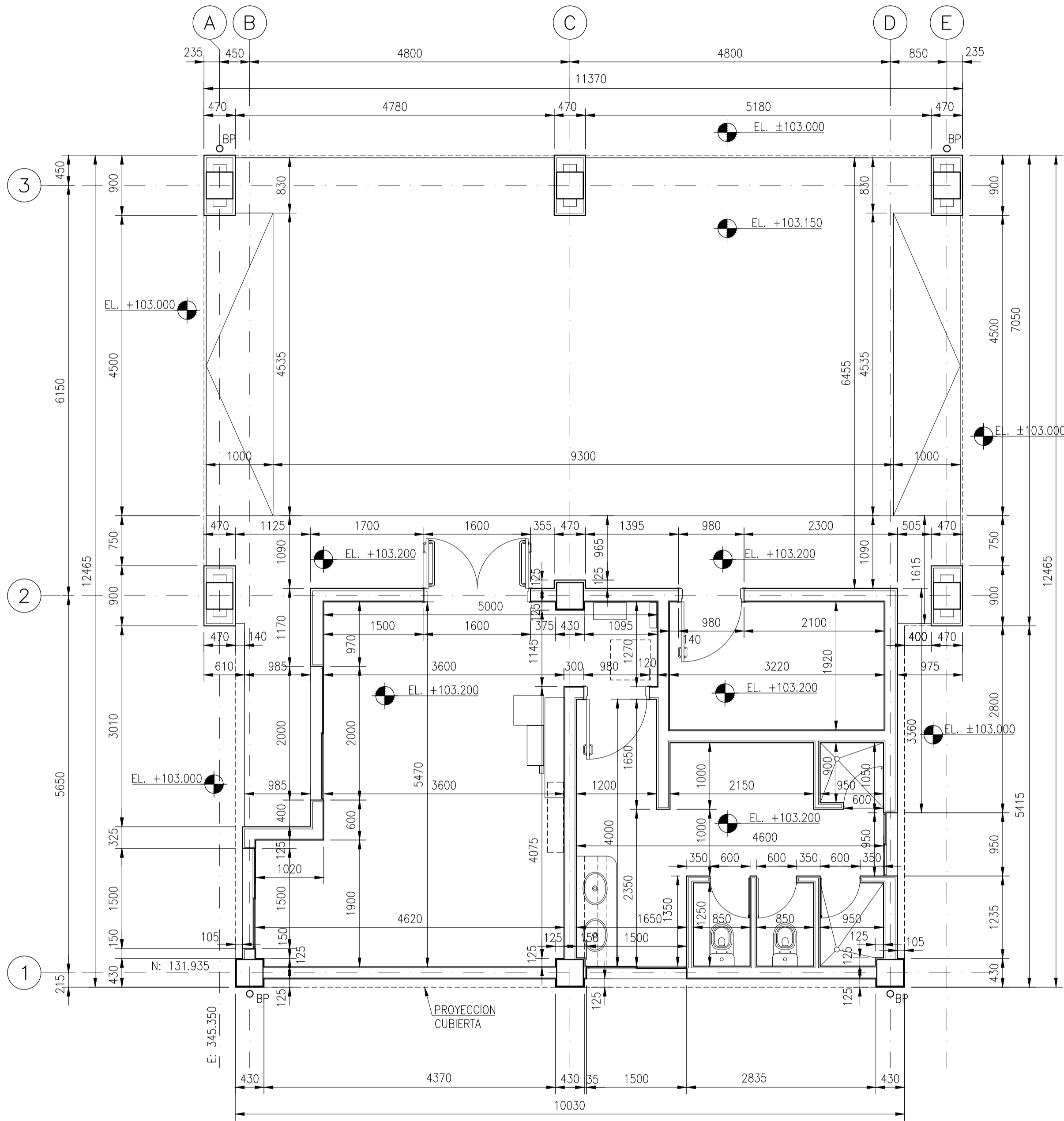
PLANTA ELEVACIÓN+103.200 ESCALA 1:50
