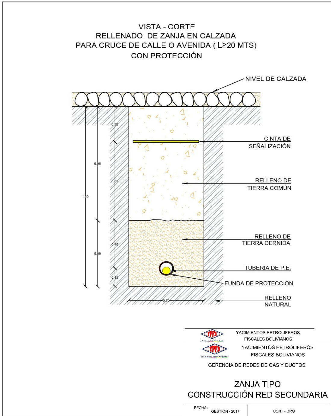
FIGURA 3.2. ZANJA TIPO CONSTRUCCIÓN RED SECUNDARIA
