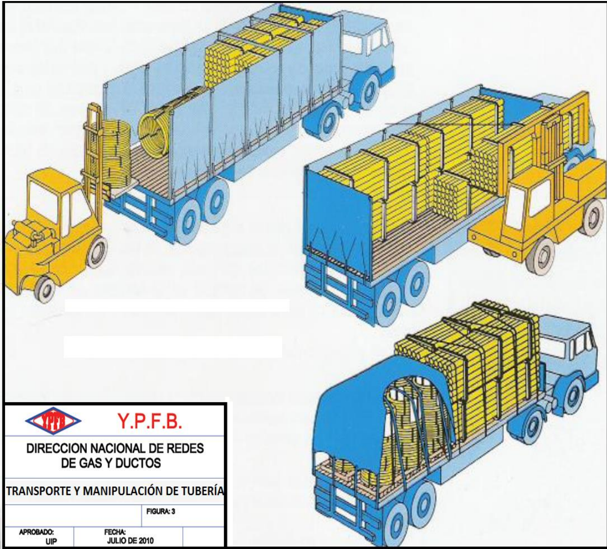
FIGURA 4. TRANSPORTE DE TUBERIA
