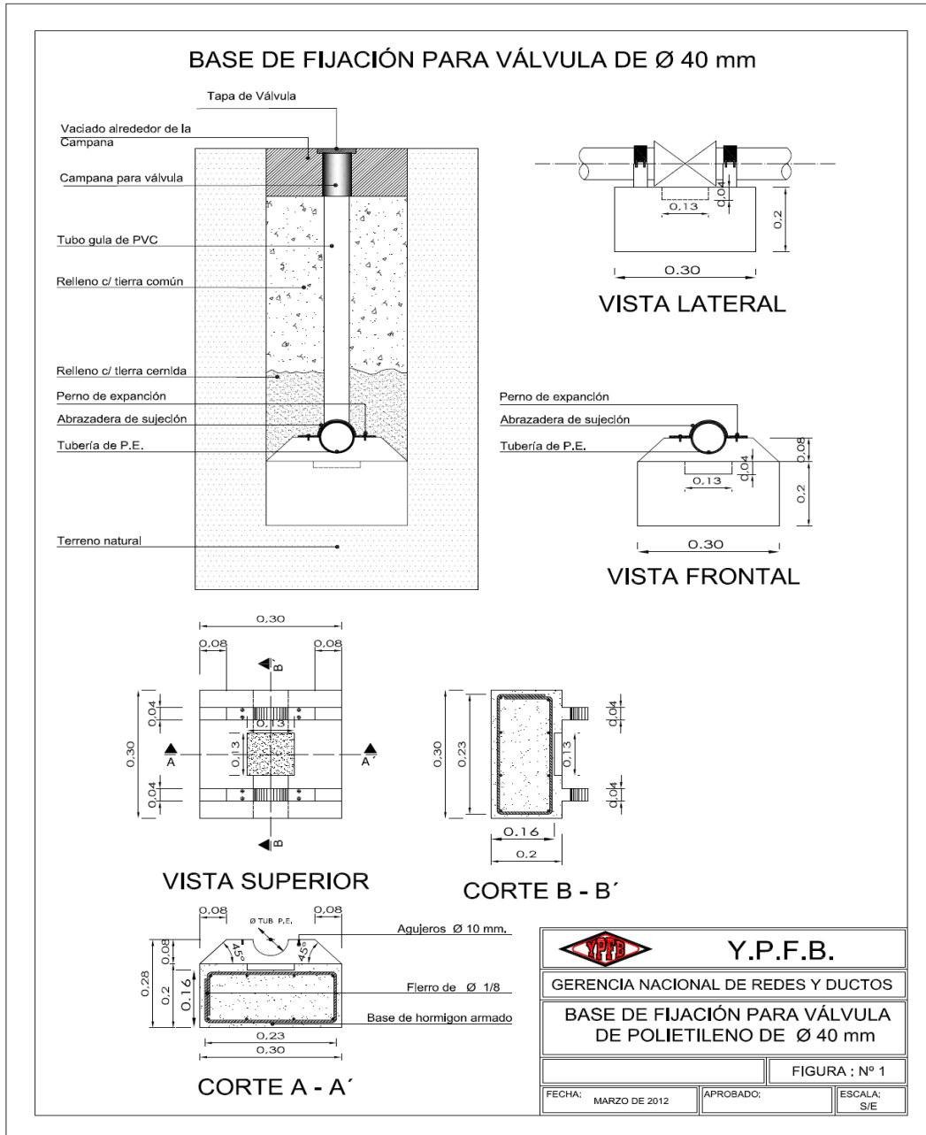
FIGURA 5. BASE DE FIJACION PARA VALVULA DE 40 mm
