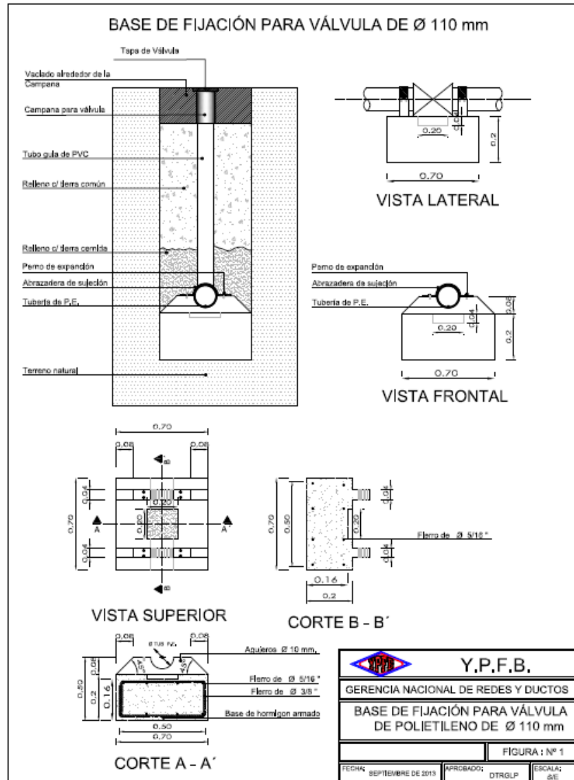
FIGURA 6. BASE DE FIJACION PARA VALVULA DE 110 mm
