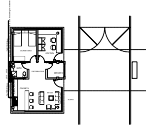
OFICINAS INSTALACIÓN DE AGUA POTABLE
