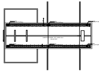
PÓRTICO INSTALACIÓN DE DESAGUE PLUVIAL
