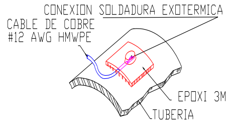
PROTECCION DE LA SOLDADURA
