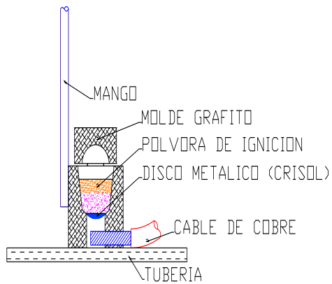
MOLDE DE GRAFITO (SOLDADURA CALDWELD)
