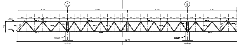
RETICULA PRINCIPAL ESC.: 1 : 50
