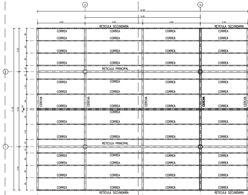
PLANTA CUBIERTA ESC.: 1 : 50
