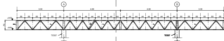
RETICULA SECUNDARIA ESC.: 1 : 50
