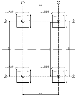
PLANTA ISLAS DE DISTRIBUCION
