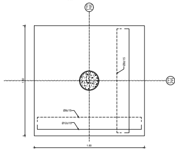
PLANTA ISLAS DE DISTRIBUCION
