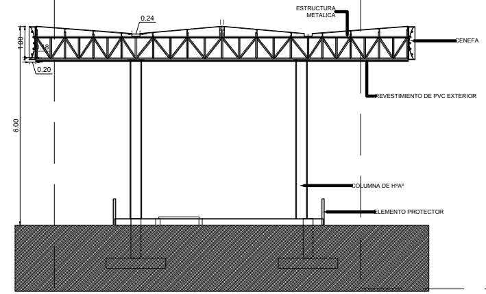
CORTE TRANSVERSAL B - B' ESC.: 1:50
