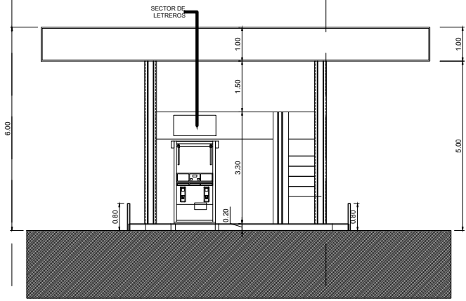
ELEVACION LATERAL SUR ESC.: 1:50
