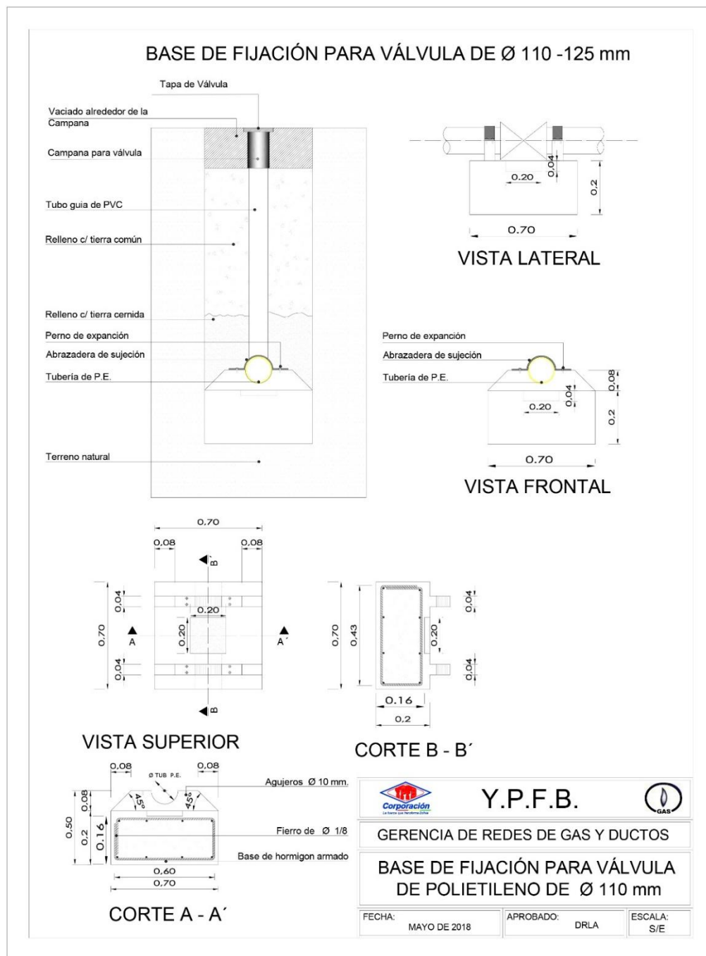
FIGURA 5.4 DETALLE DE LA BASE DE FIJACIÓN DE VÁLVULA DE P.E. 110- 125 MM
