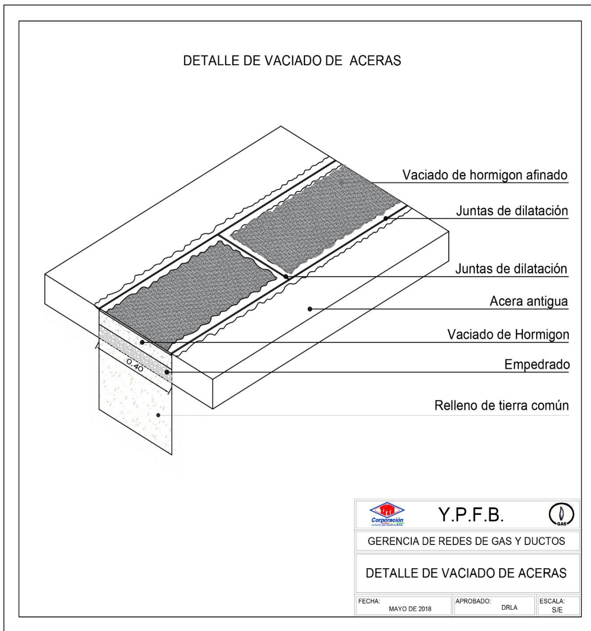
FIGURA 4.1 DETALLE DE VACIADO DE ACERAS
