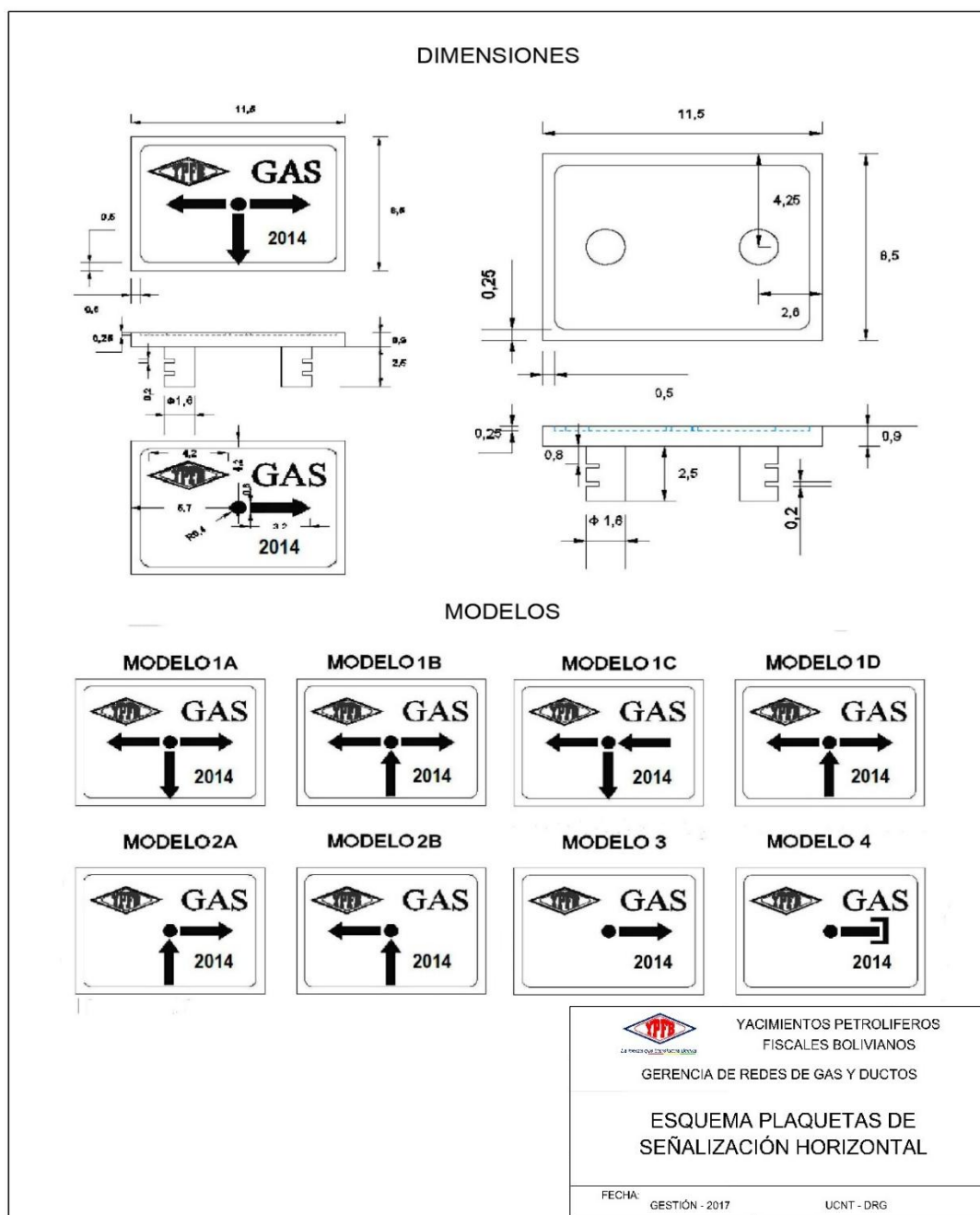
FIGURA 6. ESQUEMA PLAQUETAS DE SEÑALIZACIÓN HORIZONTAL
