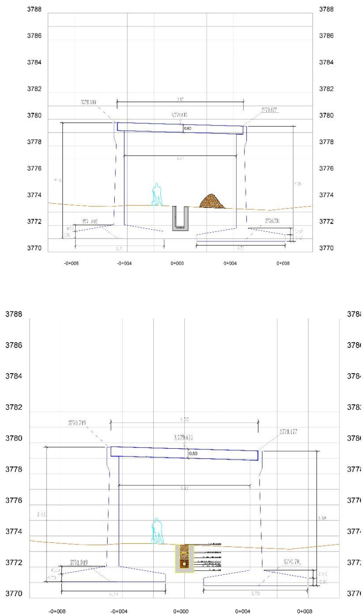
FIGURA 7.4 CRUCE 3 – VISTA DE PERFIL LATERAL IZQUIERDO
