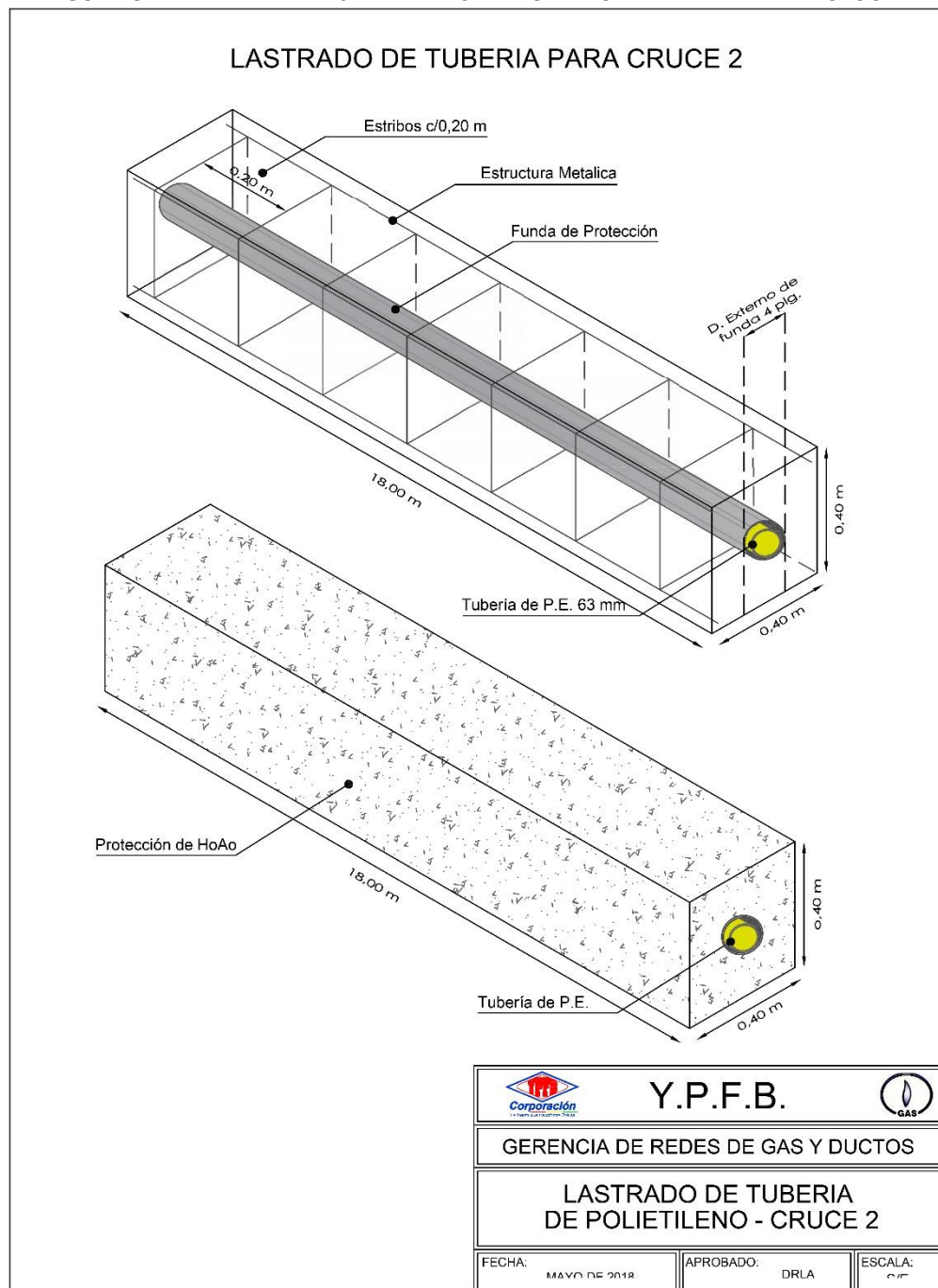
FIGURA 8.1 DETALLE DE ZANJA PARA LASTRADO DE TUBERÍA DE P.E. PARA CRUCE 2
