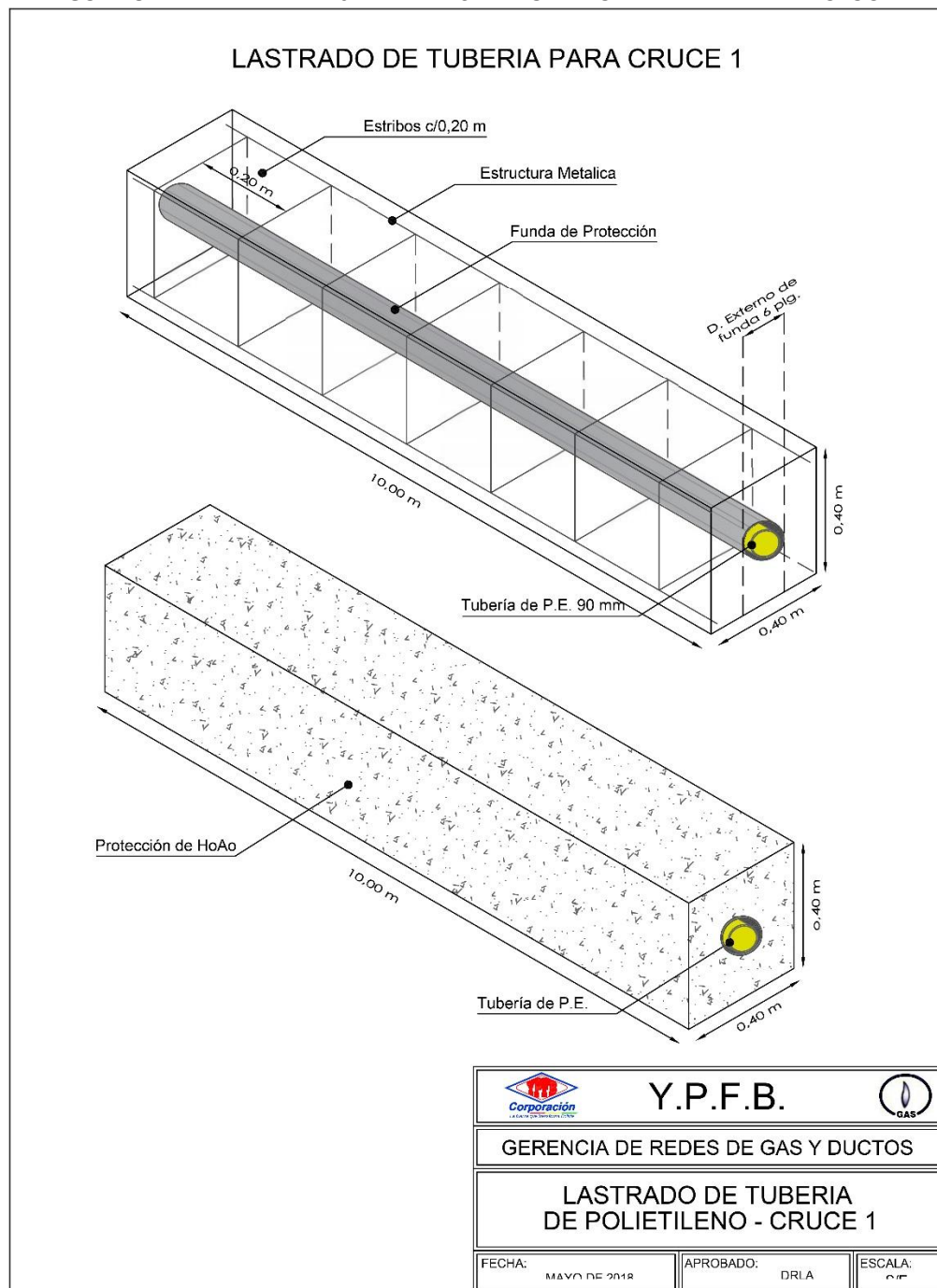
FIGURA 8.1 DETALLE DE ZANJA PARA LASTRADO DE TUBERÍA DE P.E. PARA CRUCE 1
