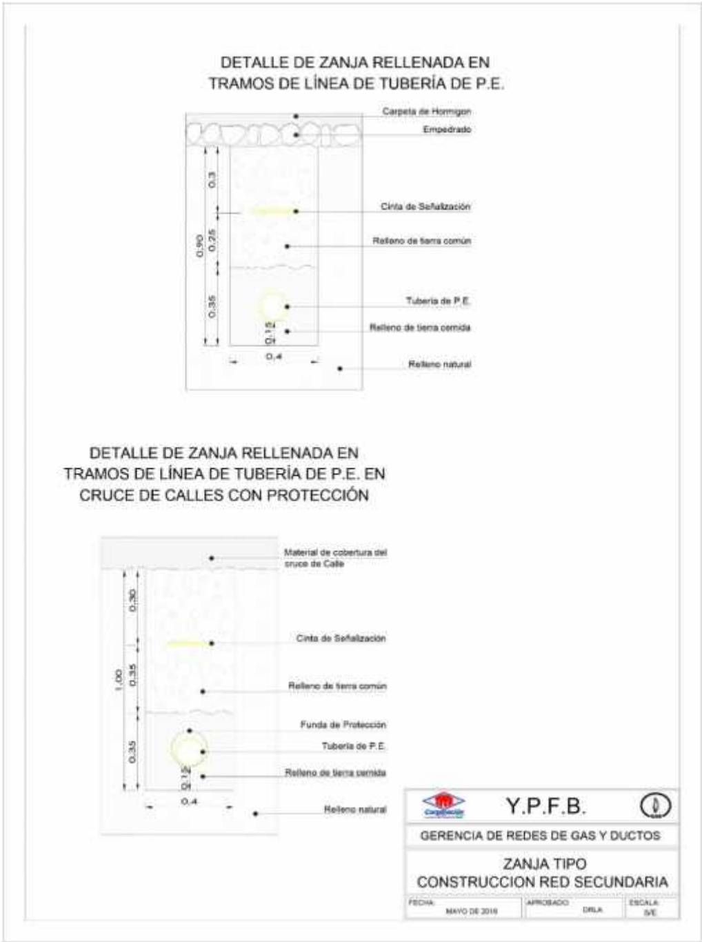
FIGURA 3. ZANJA TIPO CONSTRUCCIÓN RED SECUNDARIA
