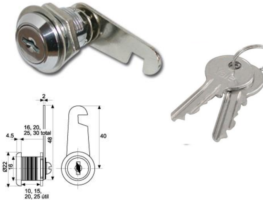
Fig. Chapa de gabinete con llave universal
